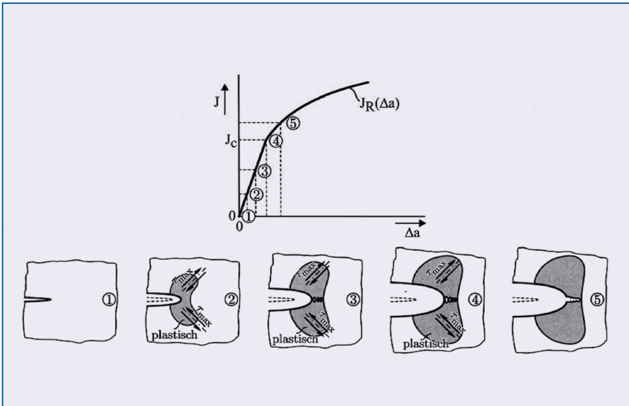
Bild 3: Was ist Blunting und wie verläuft die Rissinitiiierung?
