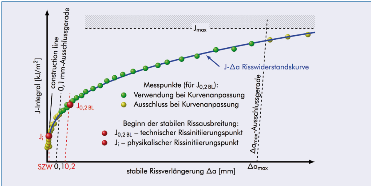
Bild 2: Rissinitiiierungspunkt
